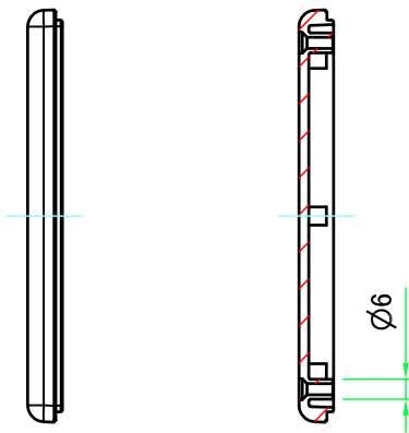
C-C ( 1 : 2.5 )
